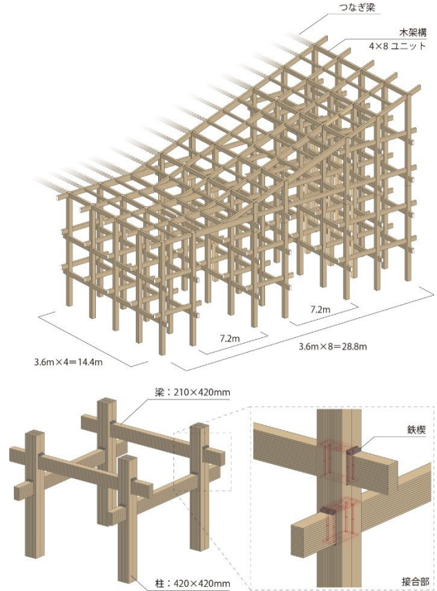
図7 木架構ユニット・接合部
